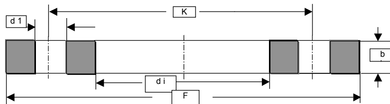
Maßliste unserer GFK-Losflansche - Anschlußmaße nach DIN 2501 ND 10
